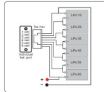
Diagramm der Balancer-Verkabelung
