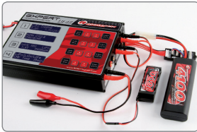
Anschluss für den Lade-, Entlade- und Storage-Modus mit Balancer
